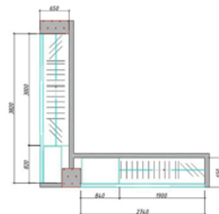
Чертежи нестандартного оборудования М 1:100
