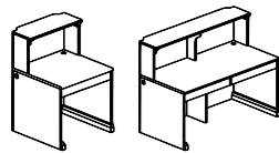
СЕКЦИЯ СТОЛА ДЛЯ ПРИЕМНОЙ [MN-RE 1] Ш: 90 / Г: 100 / В: 135 [MN-RE 2] Ш: 180 / Г: 100 / В: 135 [MN-RE 3] Ш: 270 / Г: 100 / В: 135
